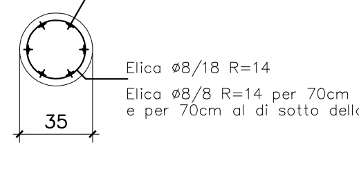
Sez. Tipo10: Pil. ø35 Pil. 17,18,19,20-1°ord
