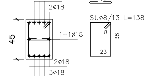
Sez. Tipo6: Pil. 30x45 Pil. n°3,4,5,6,10,11,12,13,14,15-2°&3°ord.
