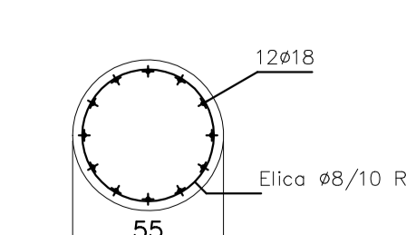
Sez. Tipo7: Pil. ø55 Pil. n°9,16-1°ord
