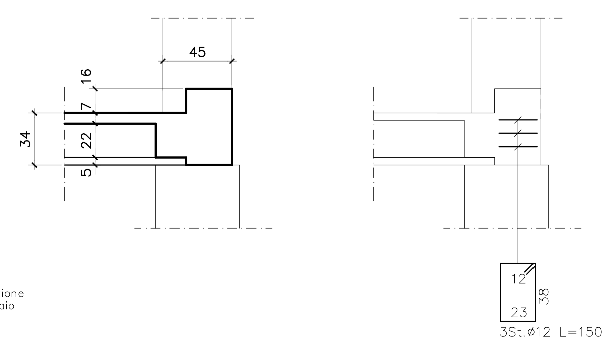
Dettaglio costruttivo nodo travi-pilastri - 1:25
