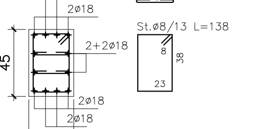
Sez. Tipo8: Pil. 30x45 Pil. n°9-2°&3°ord.
