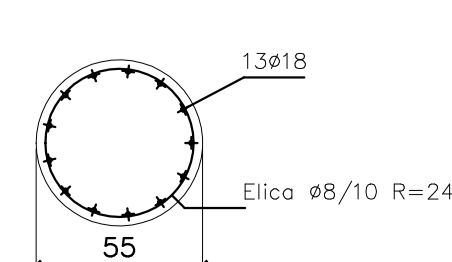
Sez. Tipo5: Pil. ø55 Pil. n°3,4,5,6,10,11,12,13,14,15-1°ord.
