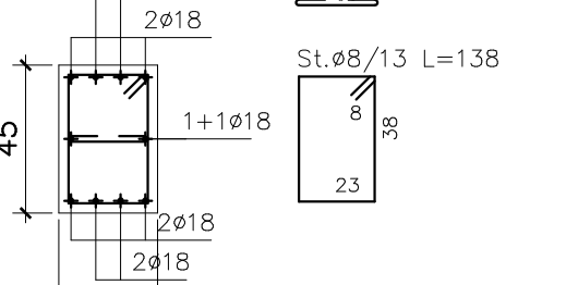
Sez. Tipo9: Pil. 30x45 Pil. n°16-2°&3°ord
