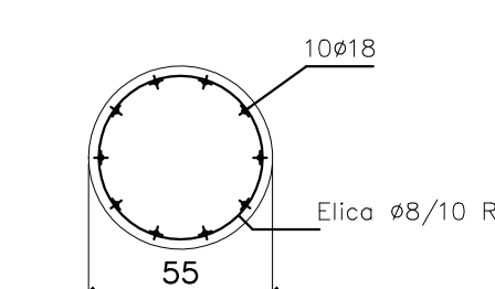
Sez. Tipo7: Pil. ø55 Pil. n°9,16-1°ord
