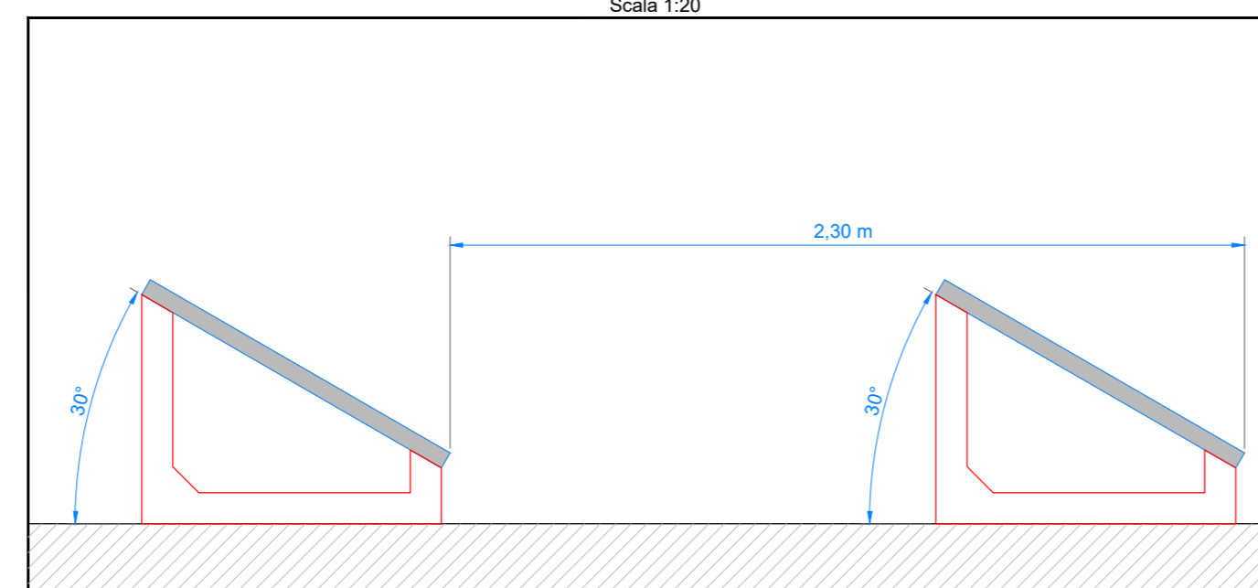
Sezione A-A' Scala 1:20
