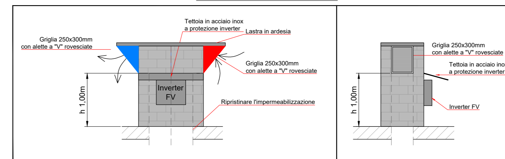
Particolare installazione inverter
